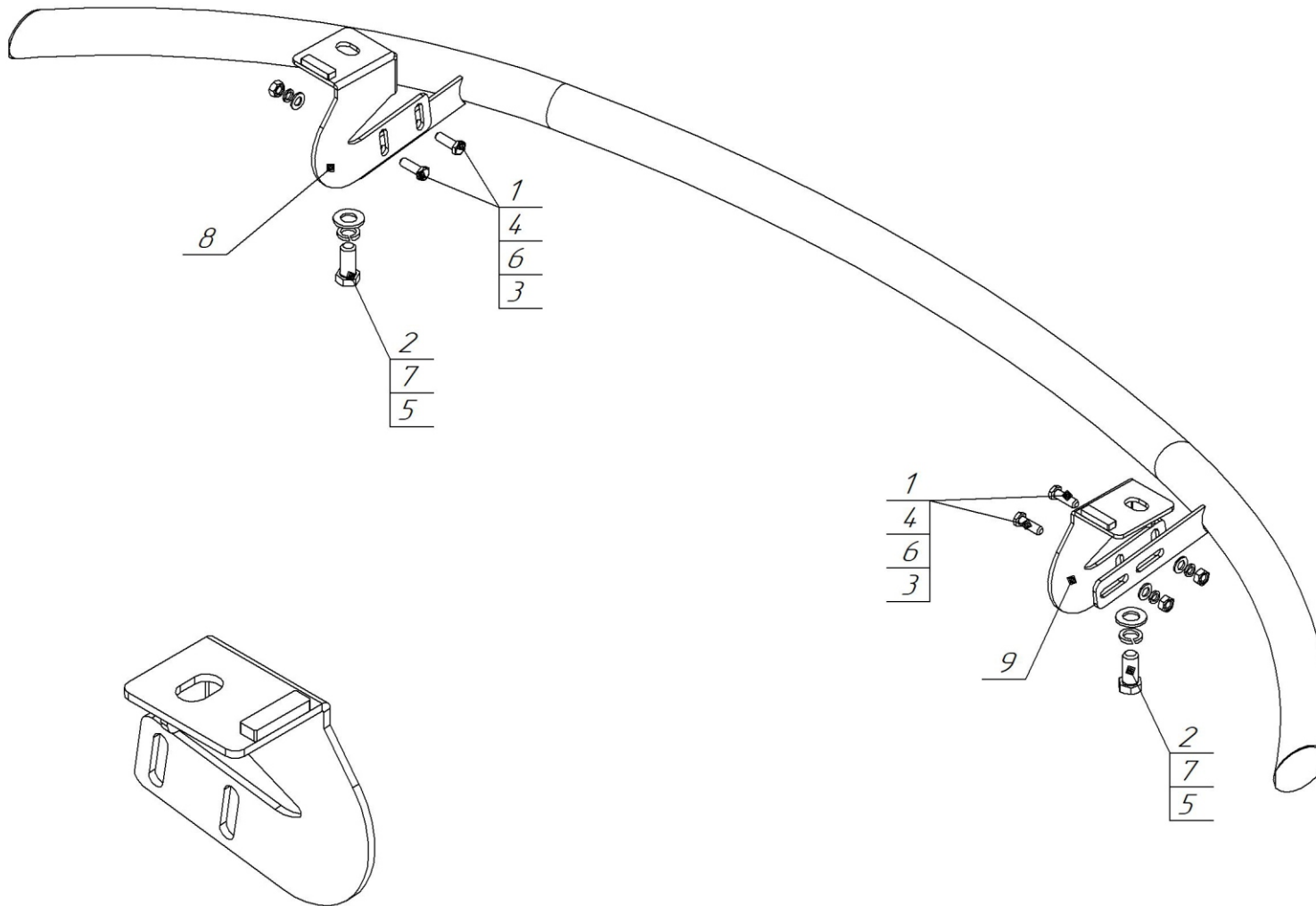
Кронштейн левый (поз.8) правый-зеркальный
